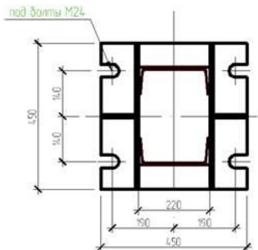
Рис.1 База колонны
