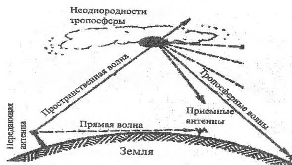
Рисунок 2 – Распространение ультракоротких волн за счет рассеяния в тропосфере
