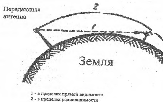
Рисунок 1 – Распространение ультракоротких волн
