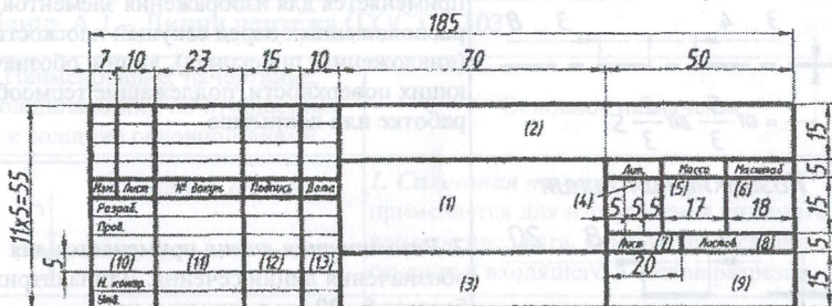
Рисунок 4.1 – Основная надпись для чертежей и схем по ГОСТ 2.104
