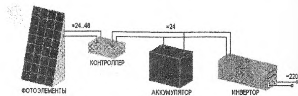
Рисунок 6 – Схема системы автономного электроснабжения на солнечных батареях
