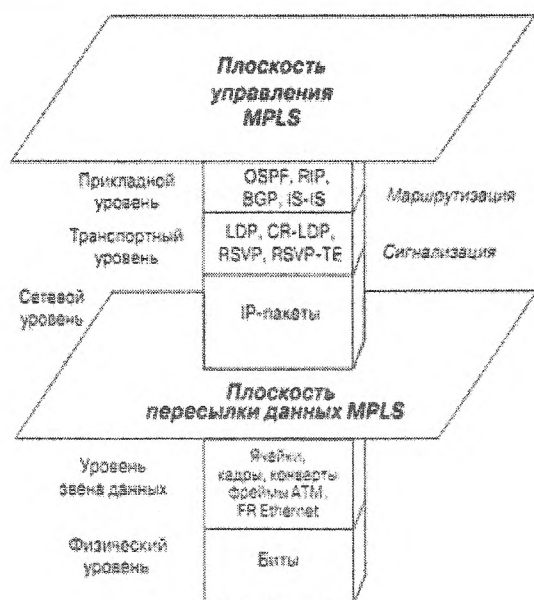
Рисунок 1 – Плоскости MPLS
