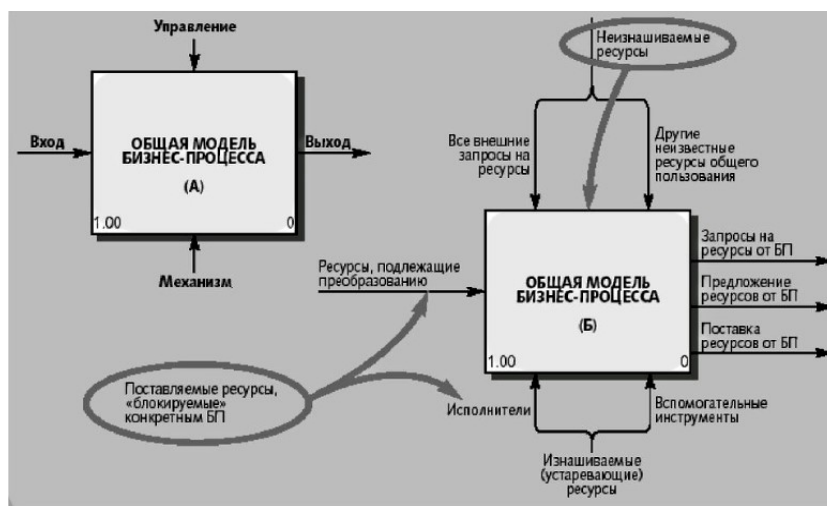
Рисунок 1 – Концепция IDEF
